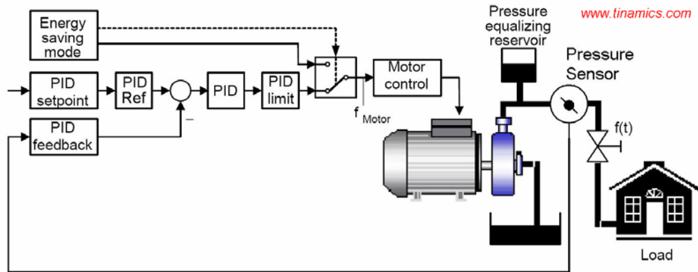
รูปที่ 3 Energy saving mode diagram
